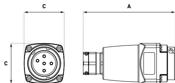
STECKER
